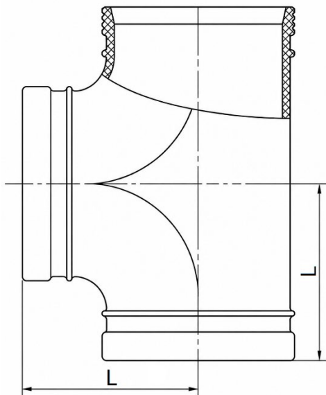
Рисунок 2 – Размеры изделия
