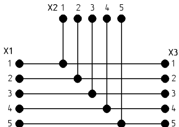
Рисунок А.2 – Схема принципиальная ПР-3
