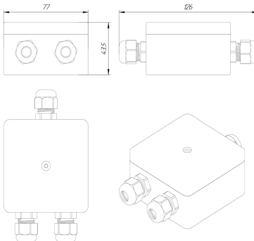
Рисунок А.1 – Габаритные и установочные размеры разветвителя интерфейса RS-422/485 ПР-3 (исполнение 2)
