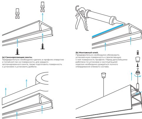
(c) Двусторонняя клейкая лента. Предварительно необходимо обезжирить установочную поверхность и прилегающую к ней поверхность профиля. Для лучшей адгезии клеевого слоя необходимо выждать рекомендованной производителем двусторонней клейкой ленты временной интервал перед дальнейшими работами по установке и эксплуатации изделия.
