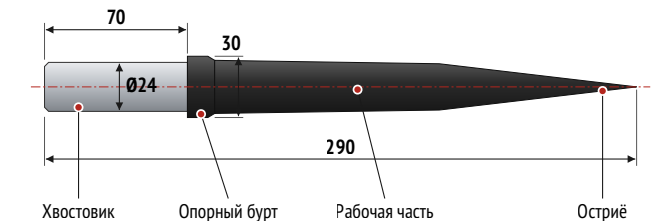
Размеры в мм. Схема приведена для пояснения устройства, масштаб условный.
