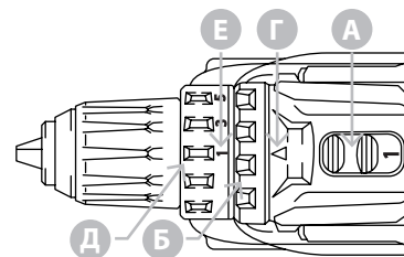
Рисунок 2.3.7. Работа в режиме шуруповёрта
