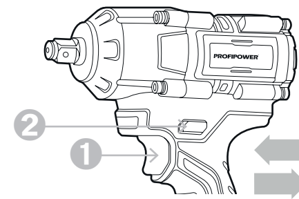
Рисунок 2.4.7. Установка направления вращения
