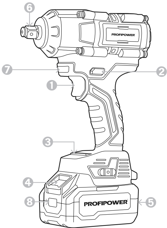
Рисунок 1.5.3. Устройство инструмента
