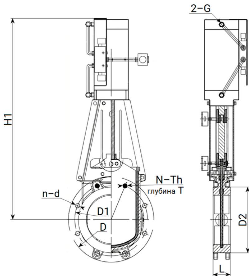
Рисунок 3 – Размеры изделия
