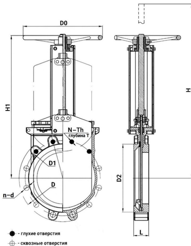
Рисунок 3 – Размеры изделия
