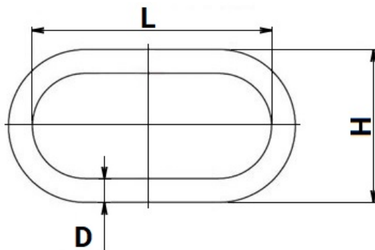
Рисунок 4 – Размеры звена цепи
