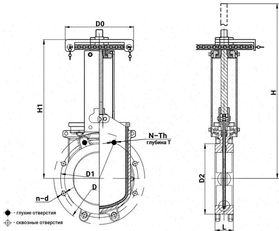
Рисунок 3 – Размеры изделия
