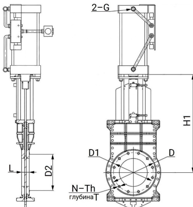
Рисунок 3 – Размеры изделия
