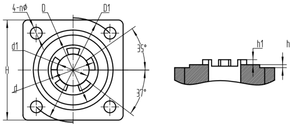
Рисунок 4 – Размеры фланца под привод
