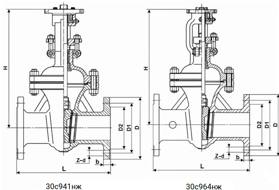
Рисунок 3 – Размеры изделия
