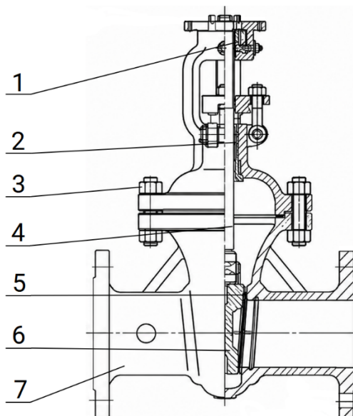
Рисунок 2 – Составные части изделия
