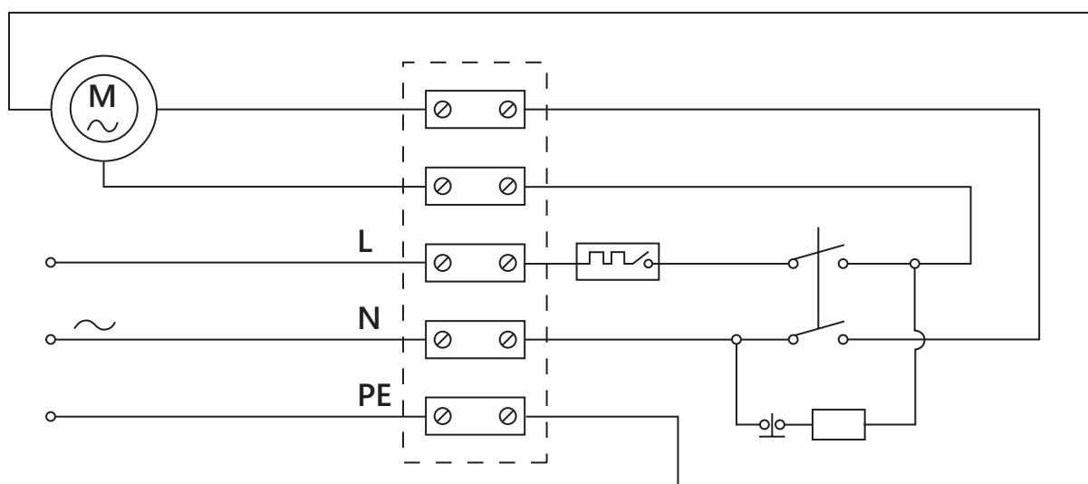
Рисунок 9. Электрическая схема для модели B0197.
