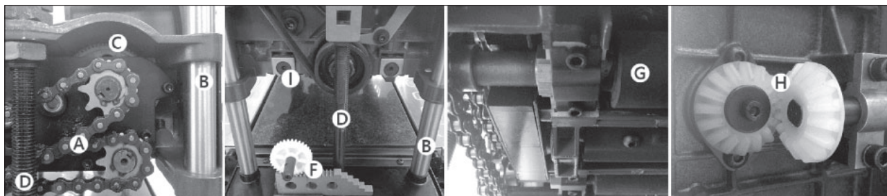
Рисунок 6. Смазка и очистка станка.
