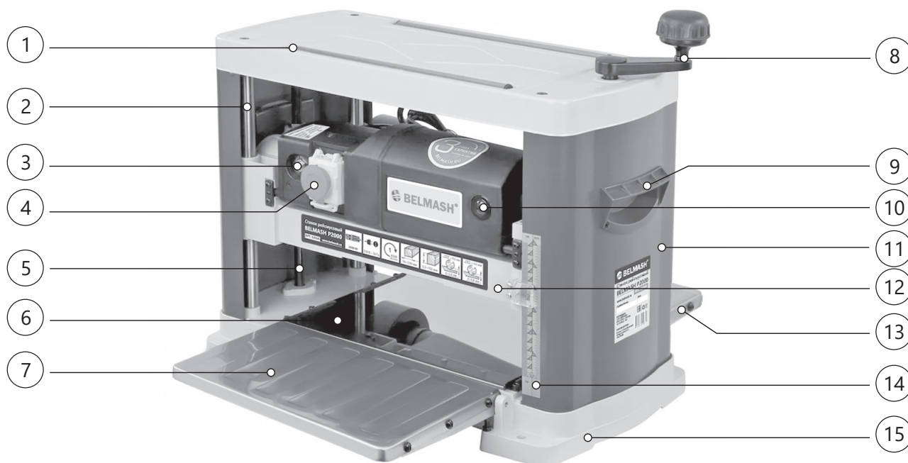
Рисунок 1. Основные элементы станка B0197.
