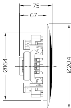
Вид сбоку
