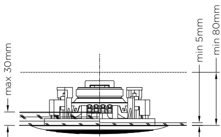
Установочные требования
