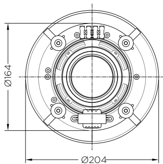
Вид снизу
