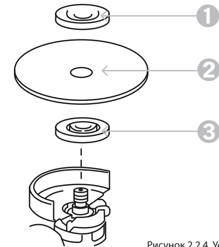
Рисунок 2.2.4. Установка оснастки
