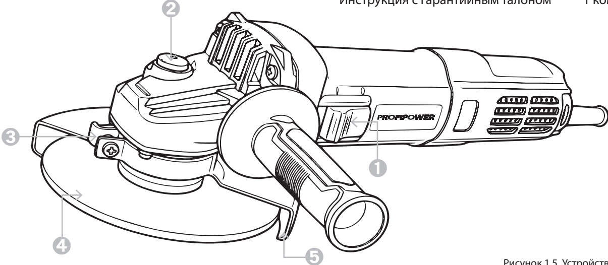
Рисунок 1.5. Устройство изделия
