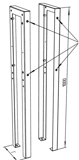
Рисунок 1. Р-образный профиль. Маркировка левой – ОНШ-Х-Х-01. Маркировка правой – ОНШ-Х-Х-02.
