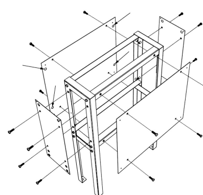
Рисунок 10. Присоединить листы к тумбе. Обратить внимание на задний лист, в котором есть дополнительные отверстия под закладные.
