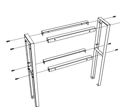
Рисунок 9. Соединить А-образные конструкции с продольными профилями, где нужно обратить внимание на положение и направление профилей.
