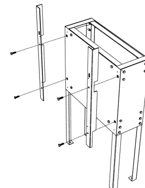
Рисунок 11. Присоединить уголки к тумбе. В дальнейшем к этим уголкам прислоняется и фиксируется задняя стенка шкафа.
