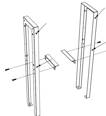
Рисунок 8. Соединить Р-образный профиль с уголками. Обратить внимание на закладные гайки в Р-образном профиле – это задняя сторона тумбы.
