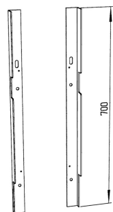
Рисунок 4. Крепление стенки. Маркировка левой – ОНШ-Х-Х-08 и правой – ОНШ-Х-Х-09.
