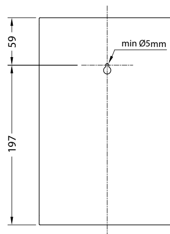
Шаблон чертежа для установки акустической системы
