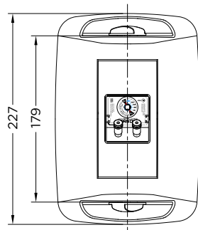
ВИД СЗАДИ / REAR VIEW
