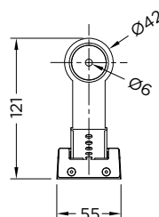
ВИД СВЕРХУ / TOP VIEW
