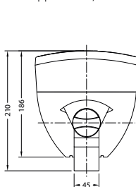
ВИД СВЕРХУ / TOP VIEW
