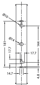
ВИД СЗАДИ / REAR VIEW
