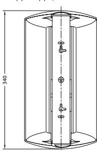
ОПЦИОНАЛЬНЫЙ ШАРНИРНЫЙ КРОНШТЕЙН SMC-65
