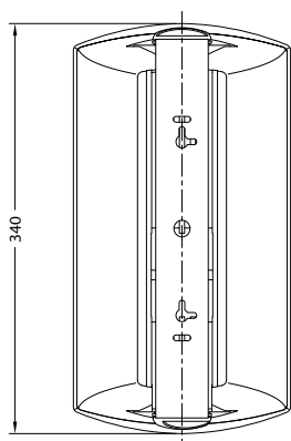
ОПЦИОНАЛЬНЫЙ ШАРНИРНЫЙ КРОНШТЕЙН SMC-65
