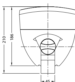
ОПЦИОНАЛЬНЫЙ ШАРНИРНЫЙ КРОНШТЕЙН SMC-65
