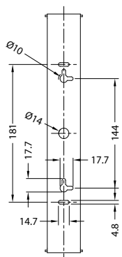
ВИД СЗАДИ / REAR VIEW
