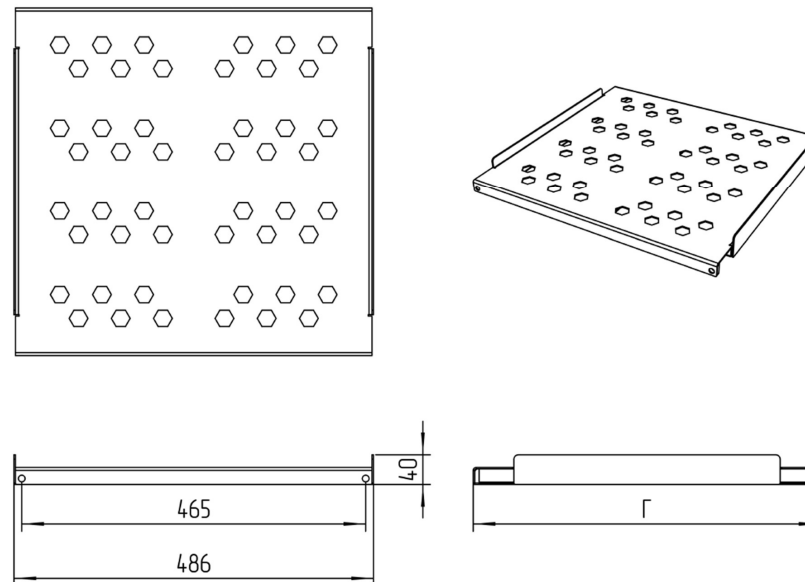
Рис. 1. Внешний вид и габаритные размеры.
