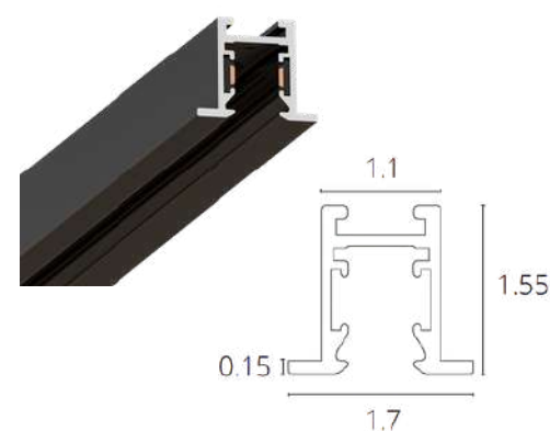
Шинопровод встраиваемый A623106 – 1 метр A623206 – 2 метра
