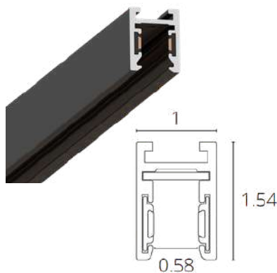
Шинопровод накладной A622106 – 1 метр A622206 – 2 метра
