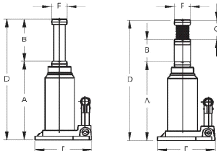
Рисунок 1. Размеры домкрата.
