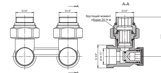
Схема 1.0020-001-D-3412
