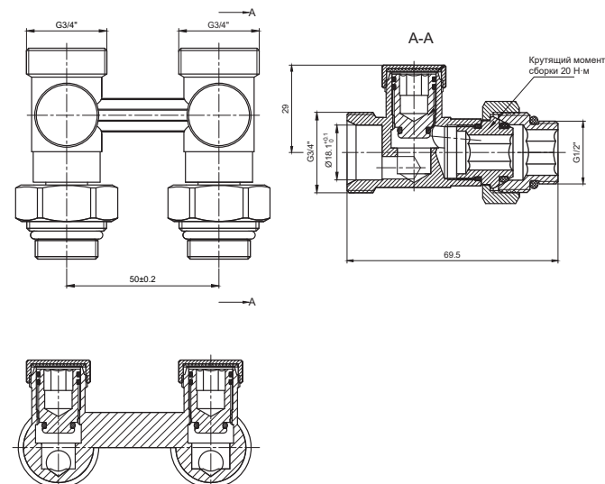
Схема 1.0020-001-D-3412
