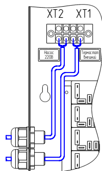
Рис.3 Схема подключения насоса и внешнего термостата
