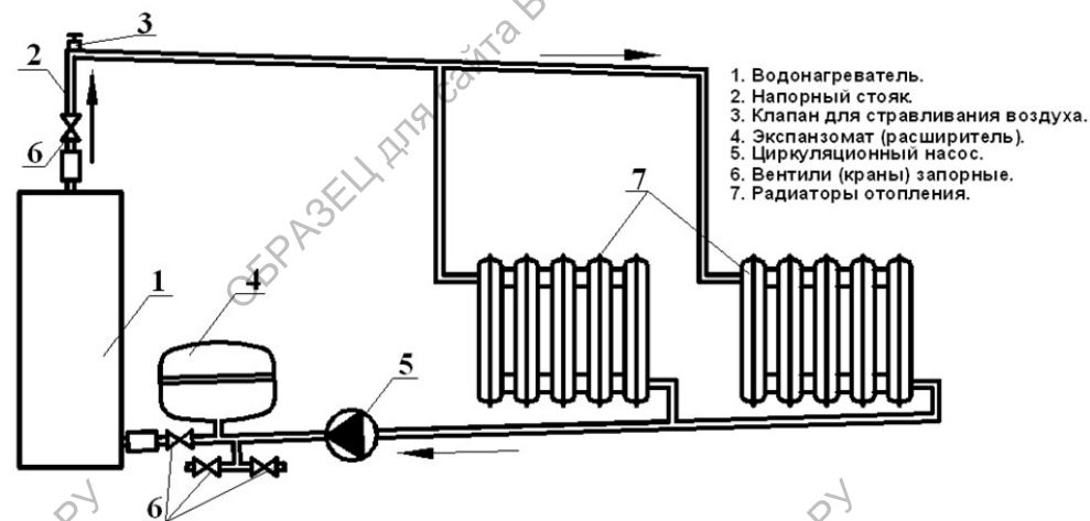
Схема включения ЭВПМ-3...12 в циркуляционную отопительную систему
