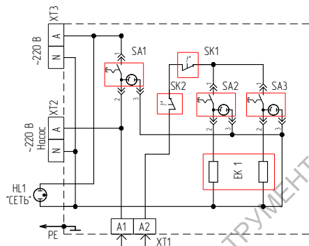
Рис.7 ЗВПМ-3 Схема электрическая принципиальная
