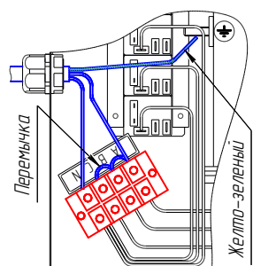
Рис.5 Схема подключения к однофазной сети ЭВПМ-4,8...9
