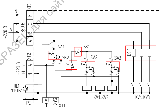
Рис.8 ЗВПМ-4, 8, 9, 0 Схема электрическая принципиальная
