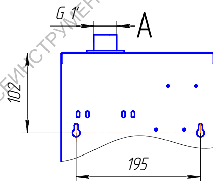
Рис.1 – Электронагреватель ЭВПМ-3...12
