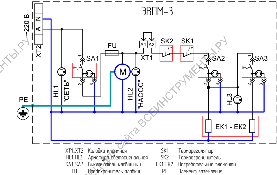
Рис.6.1 Схема электрическая принципиальная ЭВПМ-3
