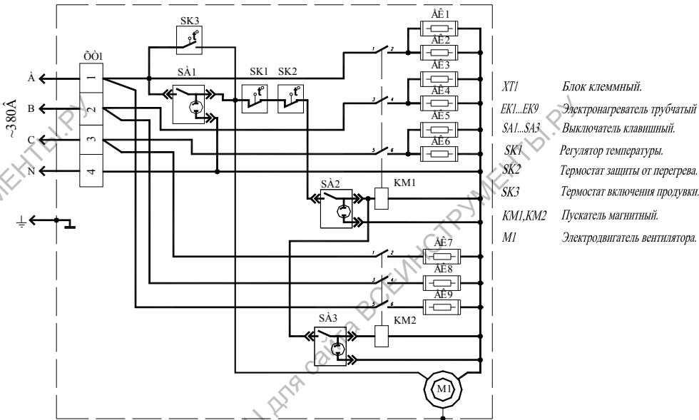
Рис.2 Калориферы КЭВ-20. Схема электрическая принципиальная..
