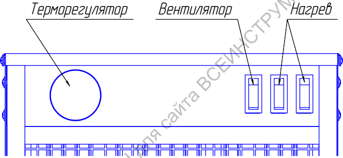
Рис. 3 – Органы управления
