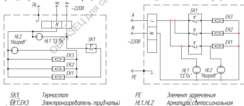
Электрокаменка ЭКМ-3
