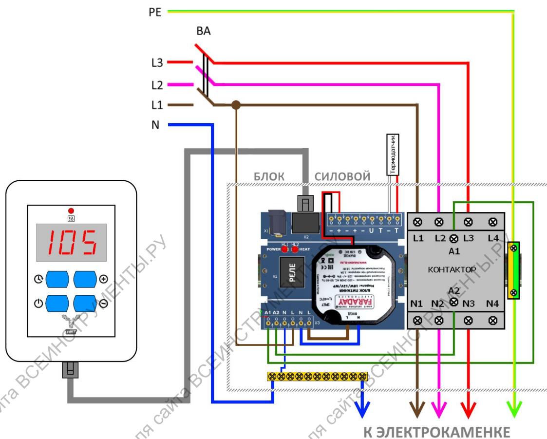
Рисунок 5. Подключение 3-х фазной каменки к пульту управления «УМТ-Лайт» 15/24/36 кВт. ↑
