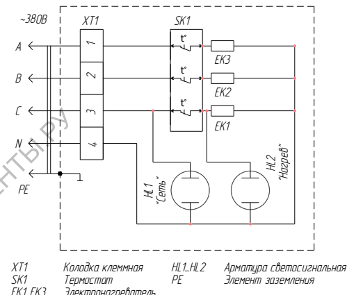
Рис.3 Схема электрическая принципиальная (слева – со встроенным терморегулятором)
