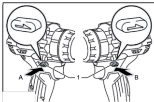
1. Переключатель хода
