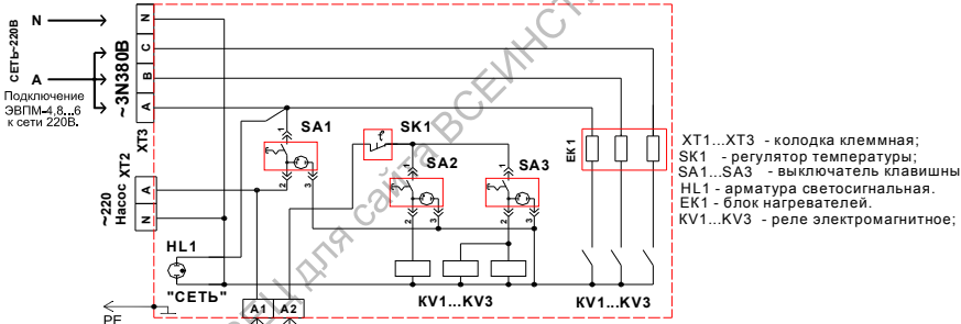
Рис. 3 ЭВПМ-4,8...12(3 реле, 3 нагревателя) Схема электрическая принципиальная.
