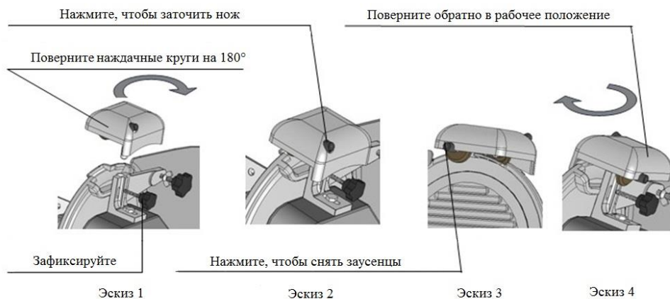
Рис.8 - заточка ножа
