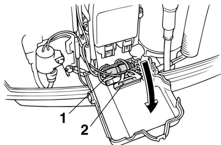
1. Держатель предохранителя 2. Плавкий предохранитель (20 A)
