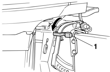
1. Рычаг фиксатора наклона
