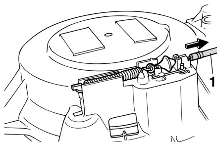
1. Трос системы защиты двигателя от случайного запуска
