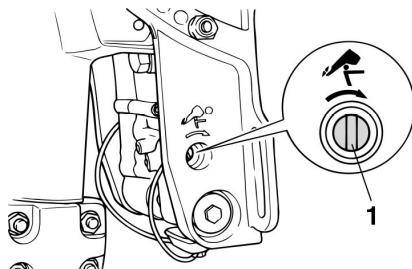
1. Винт ручного клапана
