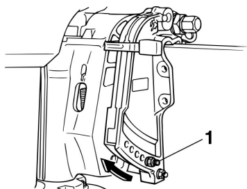
1. Тяга установки угла дифферента
