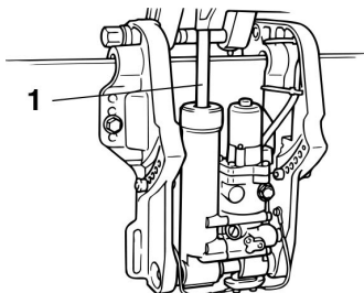
1. Тяга силового цилиндра системы наклона и дифферентовки
