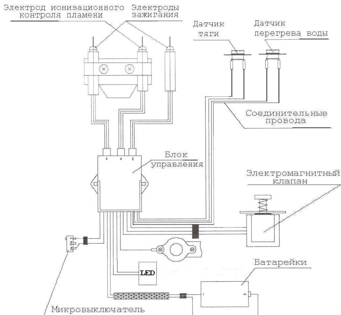
Рис. 2. Схема электрическая
