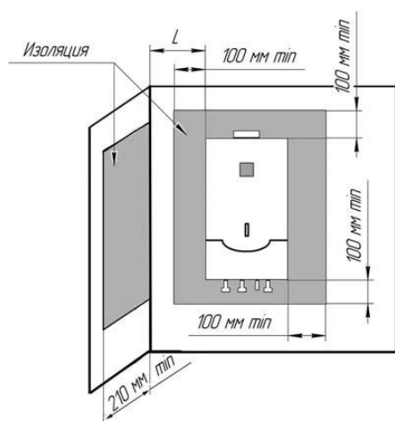
Рис. 5 Установка аппарата на трудносгораемых стенах.
