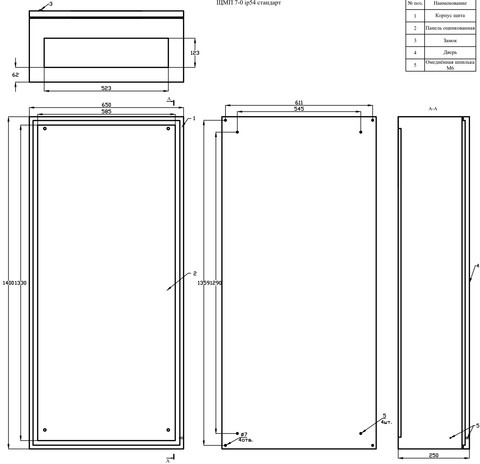
ЩМП 7-0 ip54 стандарт
