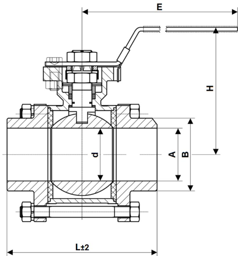
Рисунок 4 – Размеры изделия
