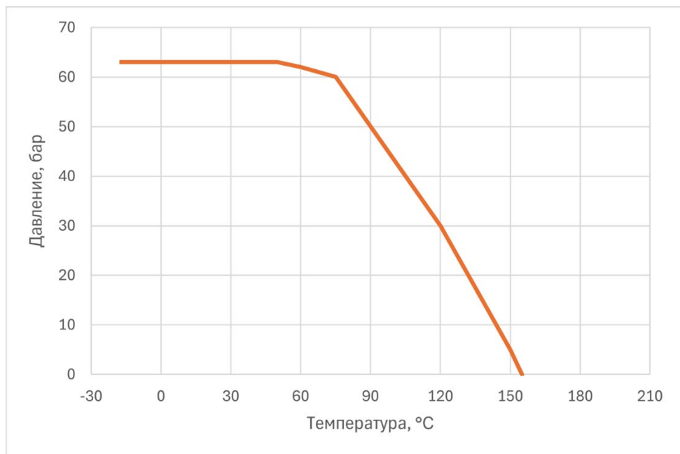
Рисунок 2 – Зависимость рабочего давления от температуры рабочей среды
