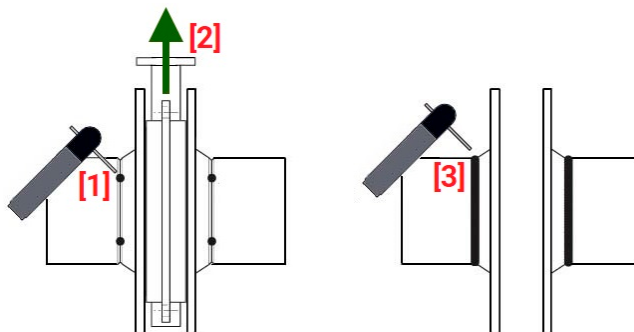
Рисунок 5 – Порядок приварки соединительных фланцев
