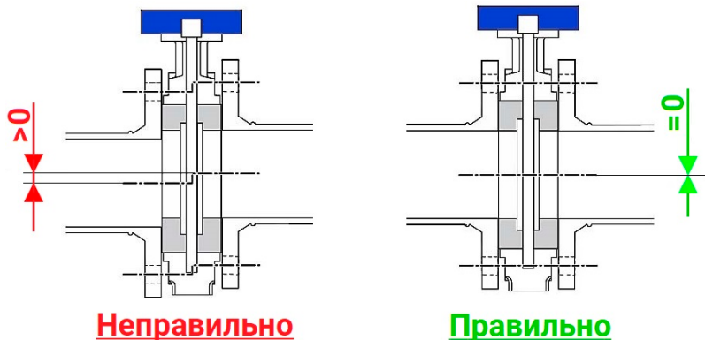
Рисунок 6 – Соосность ЗДПМ, фланцев и трубопровода
