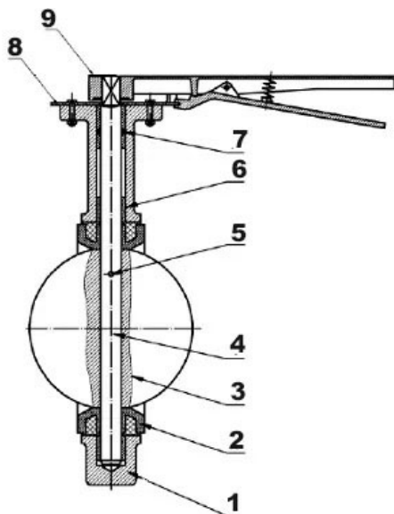
Рисунок 2 – Составные части изделия
