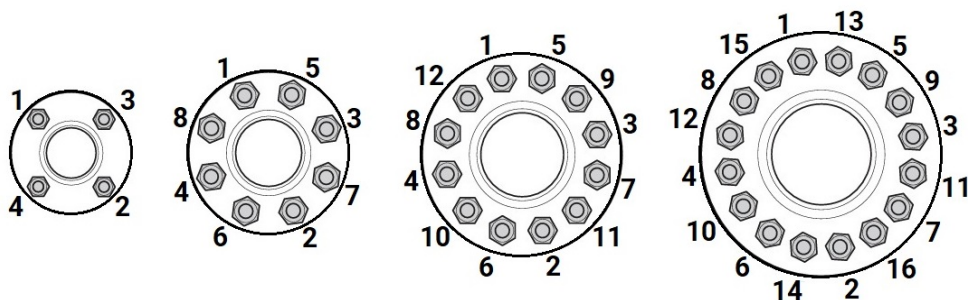
Рисунок 7 – Порядок затяжки крепежных болтов/шпилек
