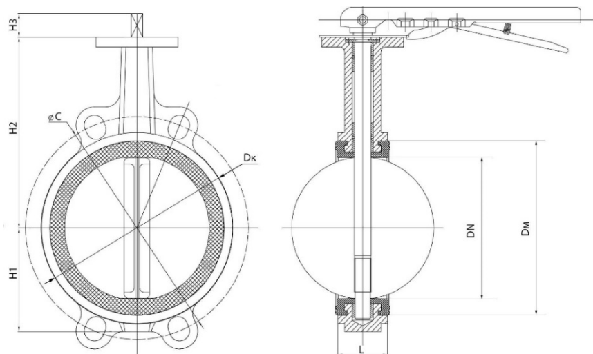
Рисунок 2 – Размеры изделия
