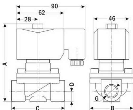
Рисунок 1. DK-2W12 Ду(12...25)
