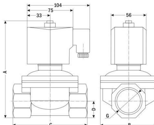
Рисунок 2. DK-2W12 Ду(32...50)
