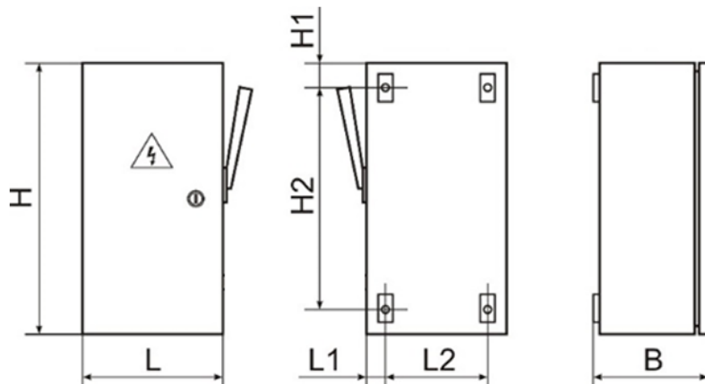
Рисунок 1. Габаритные и установочные размеры ЯРВ
