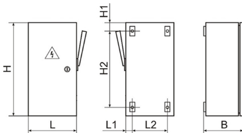
Рисунок 1. Габаритные и установочные размеры ЯРП
