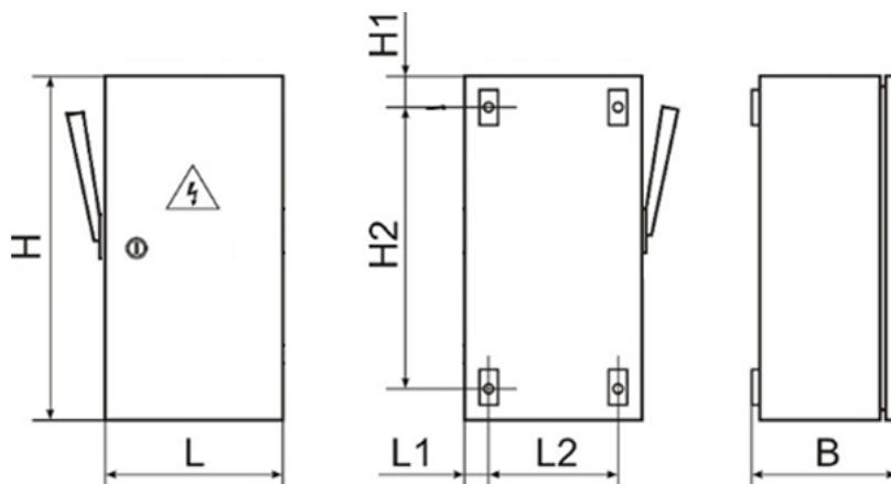
Рисунок 2. Габаритные и установочные размеры ЯРПП
