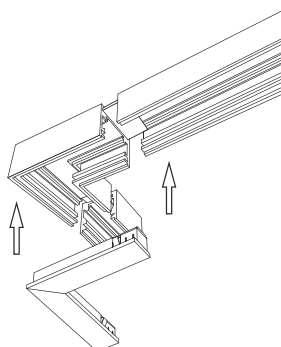
Угловое соединение шинопровода в горизонтальной плоскости
