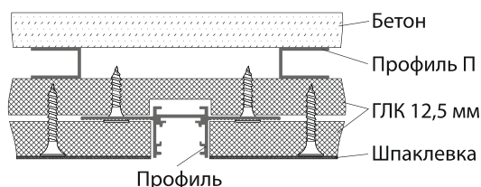
Схема монтажа шинопровода встраиваемого под ГКЛ 12,5 мм
