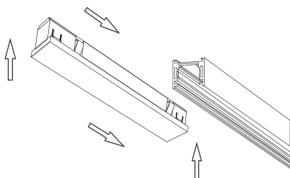
Прямое соединение шинопровода
