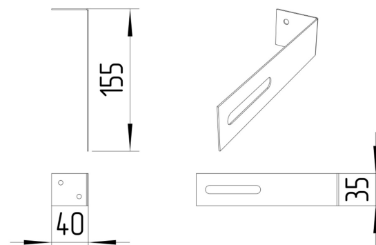
Рис. 1. Внешний вид и габаритные размеры.
