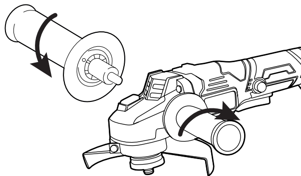
Рисунок 2.2.5. Установка боковой рукоятки
