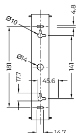
ВИД СЗАДИ / REAR VIEW
