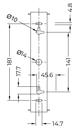
ВИД СЗАДИ / REAR VIEW
