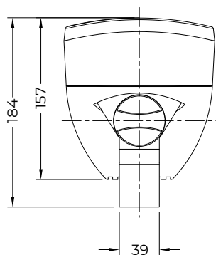
ВИД СЗАДИ / REAR VIEW
