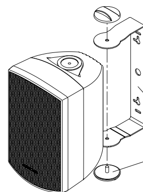
ОПЦИОНАЛЬНЫЙ ШАРНИРНЫЙ КРОНШТЕЙН SMC-65W
