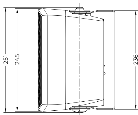
МОНТАЖНЫЙ КРОНШТЕЙН / MOUNTING BRACKET
