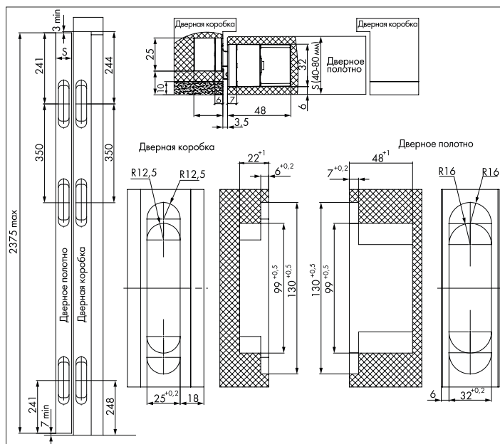
Рисунок 2 — Размеры пазов под петли.
