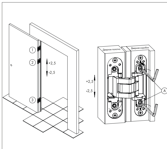
Рисунок 3 — Вертикальная регулировка.
