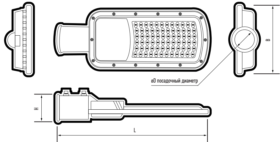
Рис.1 Габаритные размеры светильника PSL 07
