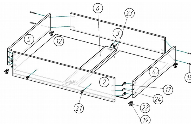
Рис.4 Сборка ящика
