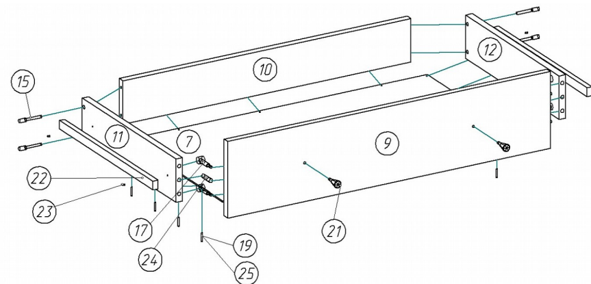
Рис.3 Установка эксцентриковой стяжки
