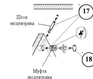
Рис.3 Установка эксцентриковой стяжки
