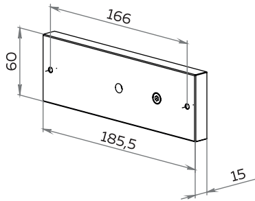
поз. 4 – Ответная планка
