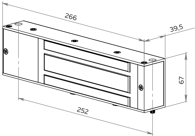
поз. 1 – Электромагнит
