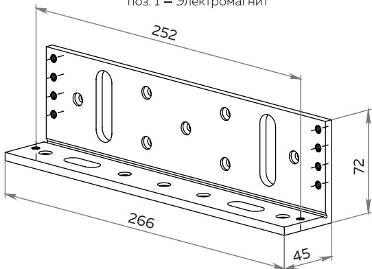
поз. 3 – Монтажный уголок
